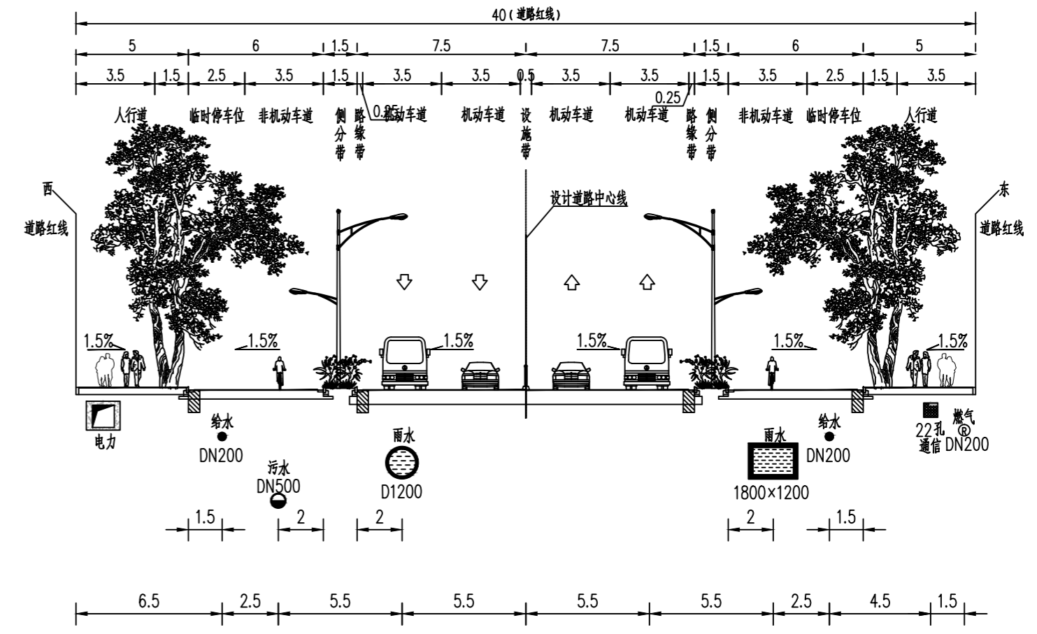
南沙路北段管综横断面
