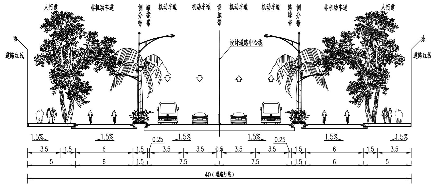
南沙路北段标准横断面
